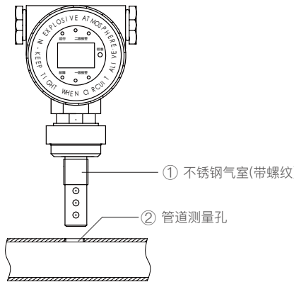
管道插入式安装示意图
