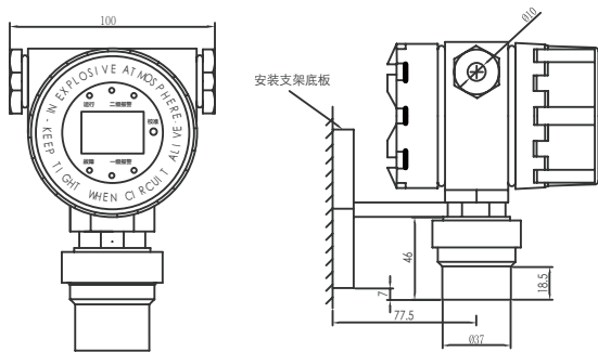
探测器壁挂式安装示意图
